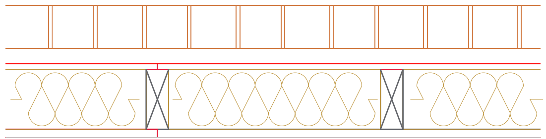
Horizontalschnitt; 1:20
