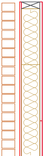
Vertikalschnitt; 1:20
