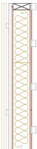
Vertikalschnitt; 1:20
