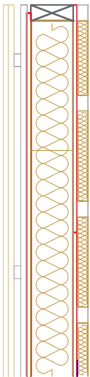
Vertikalschnitt; 1:20
