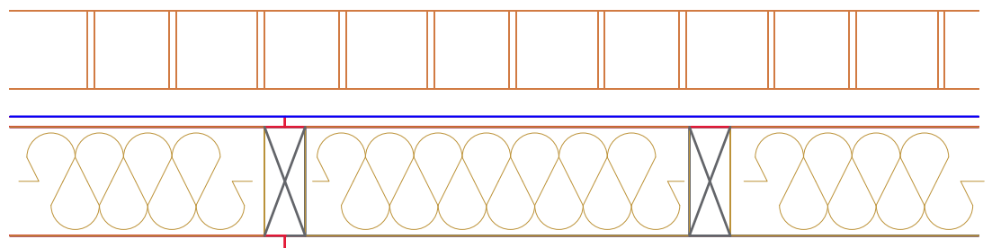
Horizontalschnitt; 1:20
