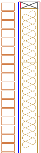
Vertikalschnitt; 1:20
