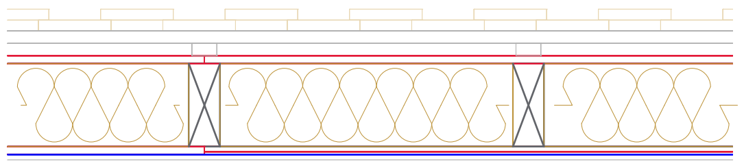
Horizontalschnitt; 1:10
