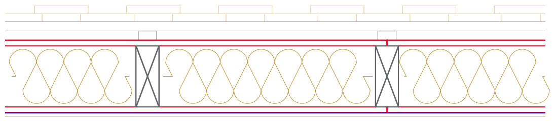
Horizontalschnitt; 1:10
