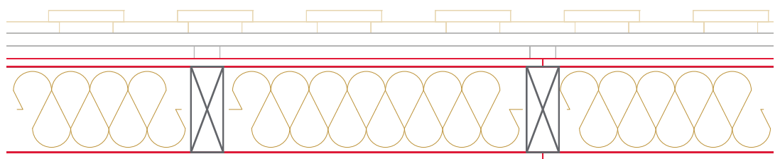
Horizontalschnitt; 1:10
